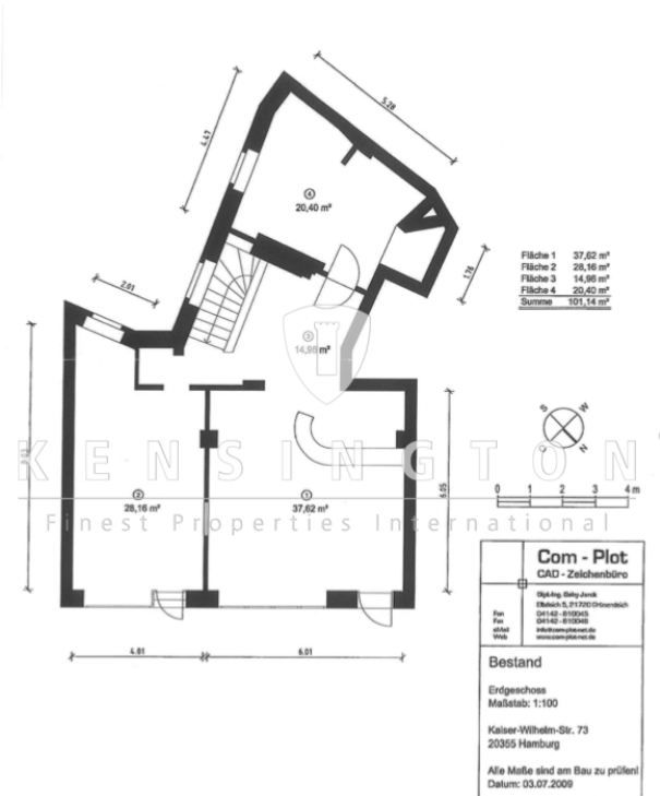
Grundriss EG
